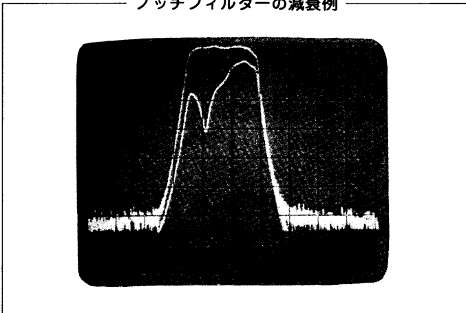
ノッチフィルターの減衰例
